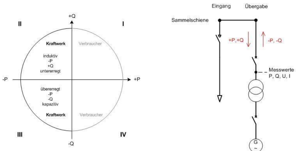
Bild 2: Verbraucherzählpeilsystem: Bezugspunkt Sammelschiene der Schaltanlage
